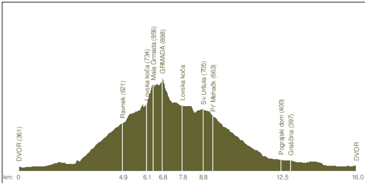
Profil poti
