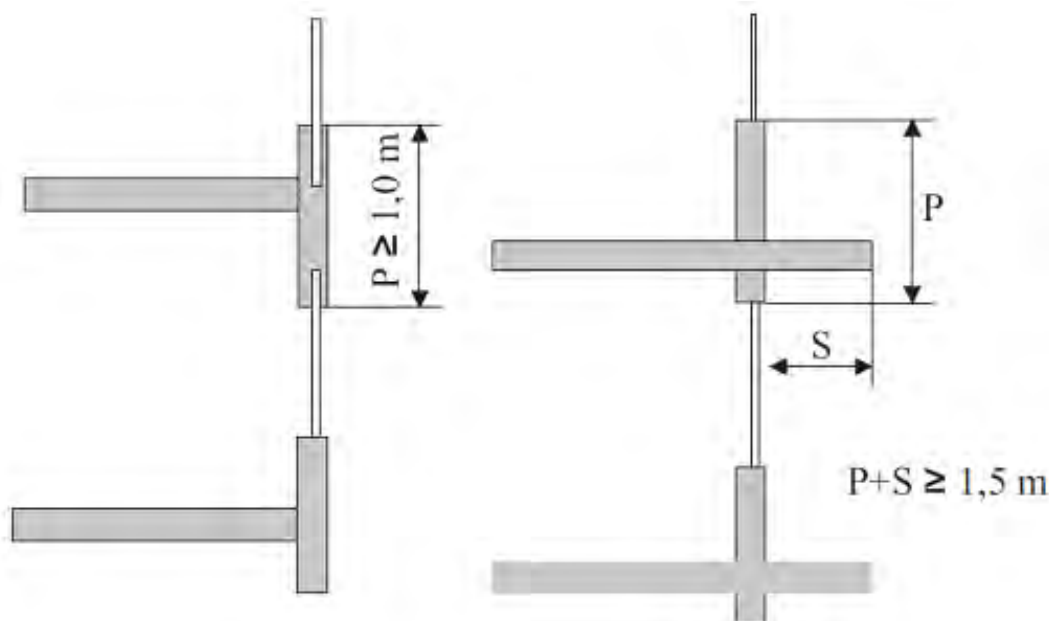
Slika 2.1: vertikalni razmik med okni v zunanji steni
