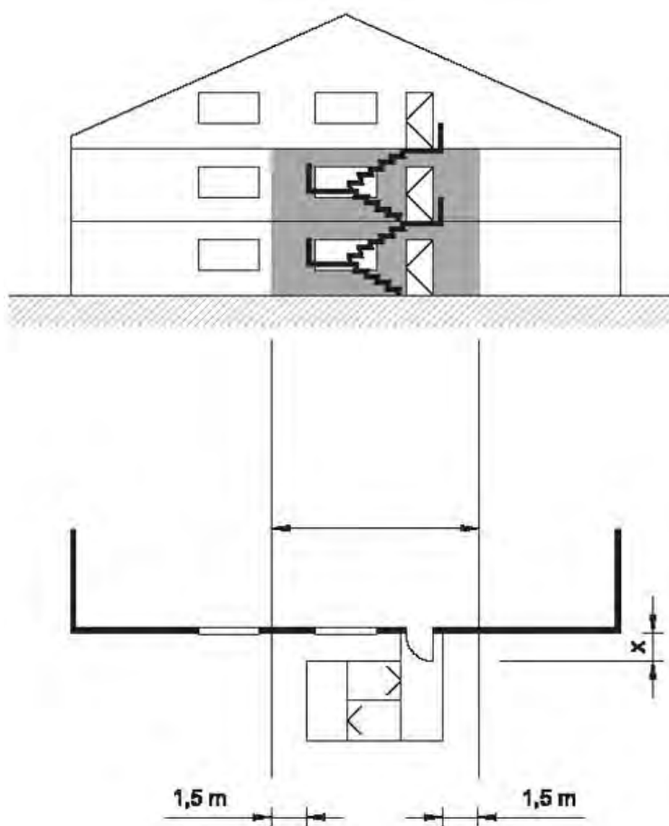
Slika 3.2: prikaz izvedbe zunanjega stopnišča
