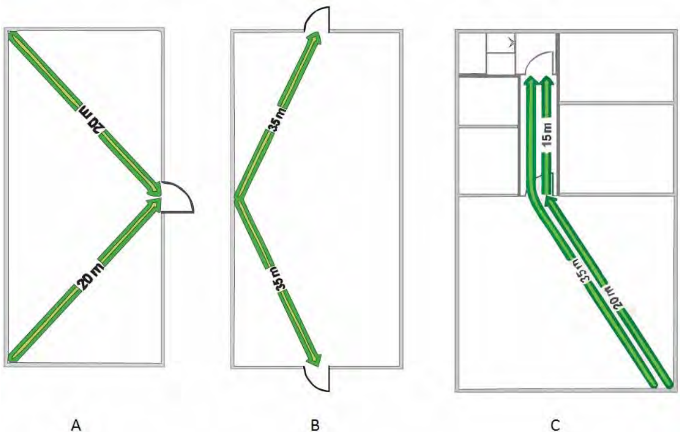
Slika 3.1: Maksimalne dolžine do izhoda:
